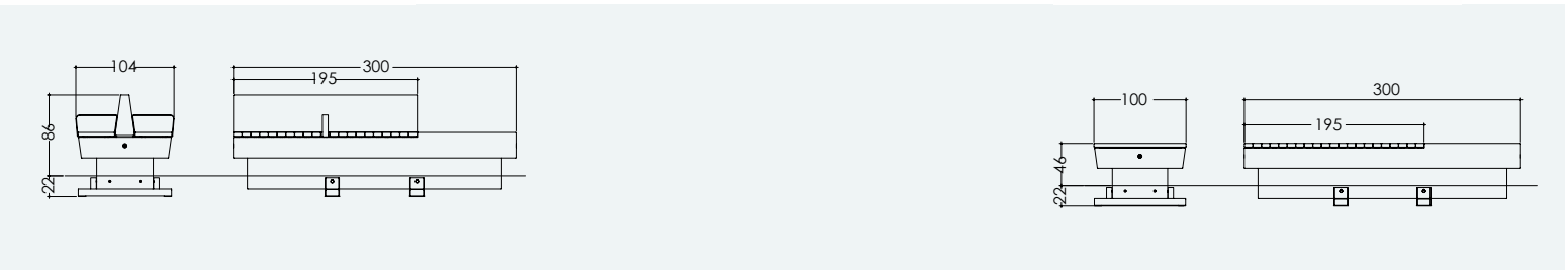
אופציה לקרקע משופעת עד 4%
