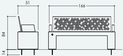
1076 ספסל נגב, בטון עם משענת מתכת ומסעד יד, נגיש, בטון, אפור
