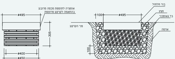
2958 בור חלחול פלסטי עם מכסה
